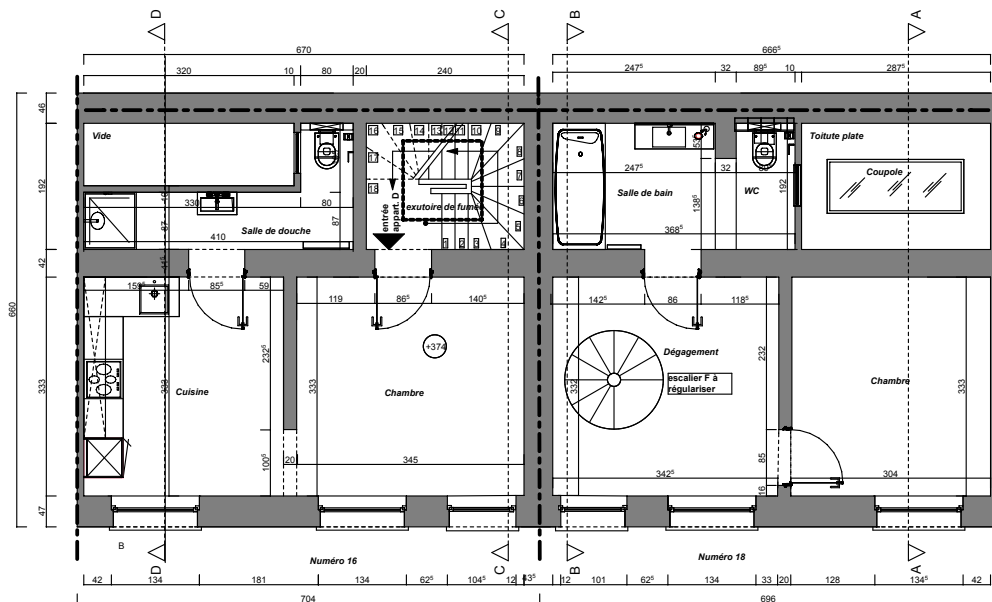
Niveau +2
