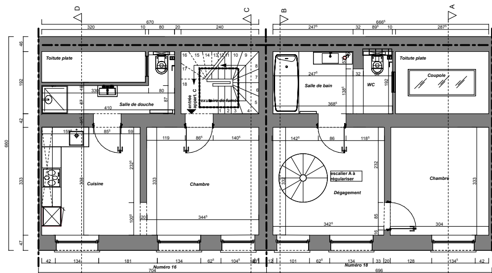
Niveau +1
