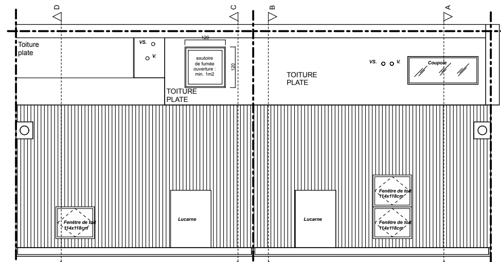
Toiture
