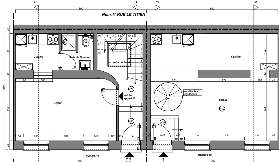
Niveau +1
