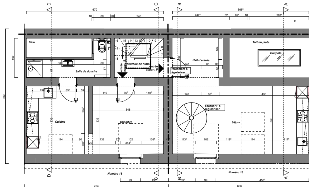
Niveau +3
